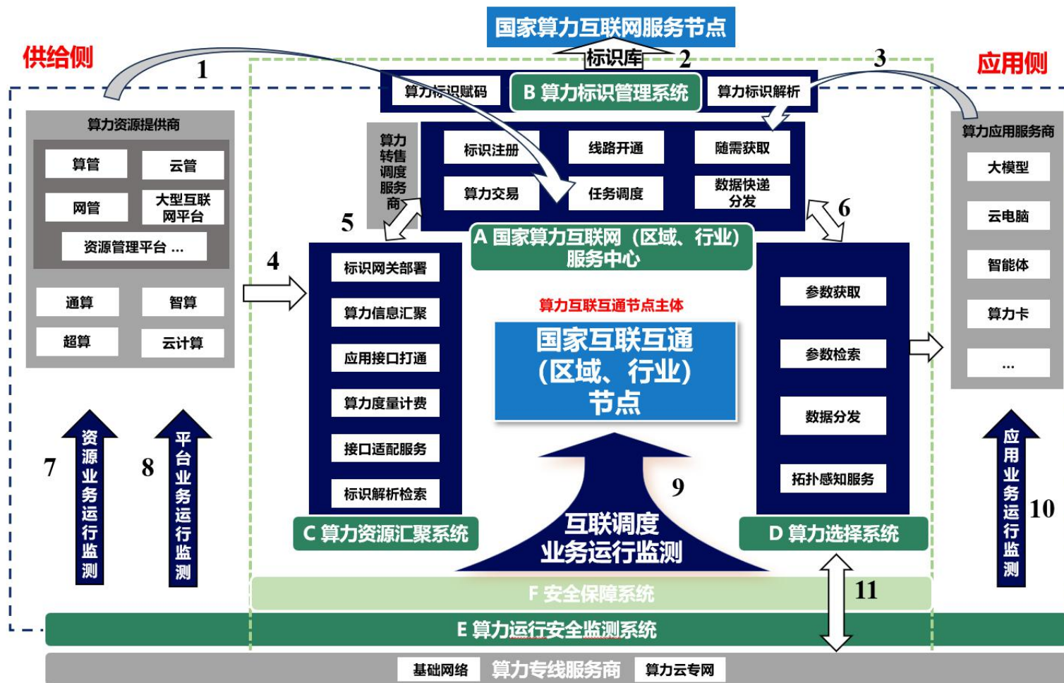
图2：国家算力互联互通（区域、行业）节点示意图
